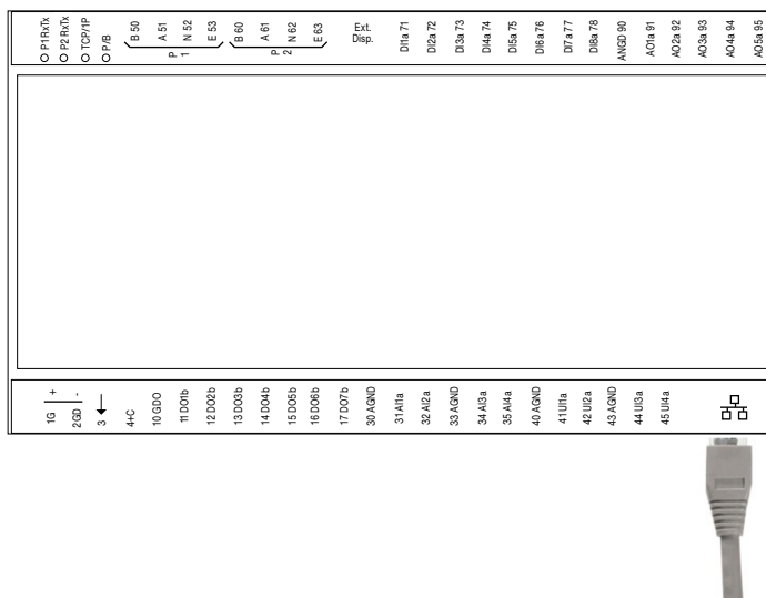
Raccordement du câble Ethernet RJ45 sur le port IP du régulateur
