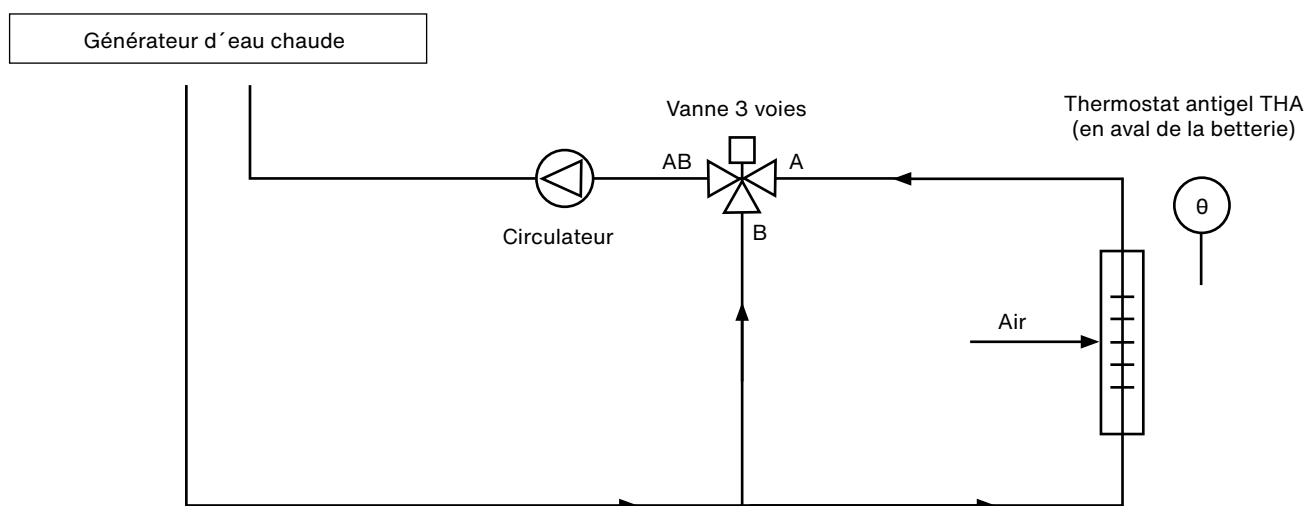
Principe de raccordement de la batterie d'eau chaude intégrée
