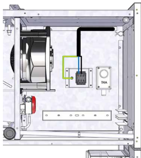
Raccordement de l'alimentation électrique sur l'interrupteur sectionneur
