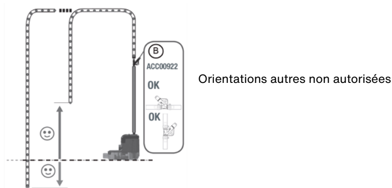
Préconisations de montage du dispositif anti-siphonnage
