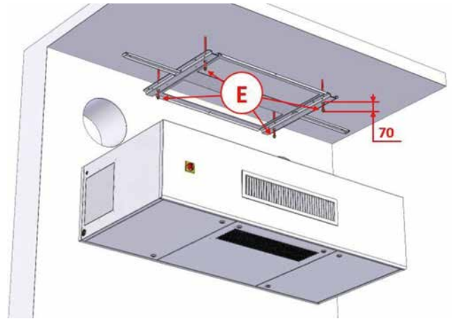
(B) Montage décalé du plafond
