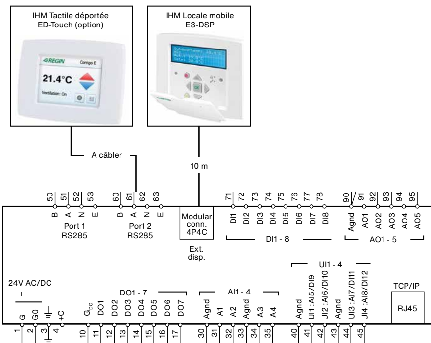
Raccordement électrique des IHM livrées de série (E3-DSP-CLD) et optionnelle (Zehnder ED-Touch)
