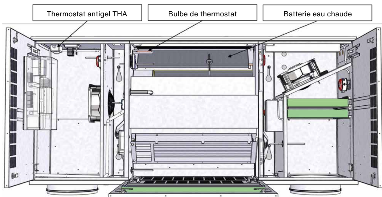
Localisation du thermostat antigel THA et de son bulbe (centrale vue de dessus)
