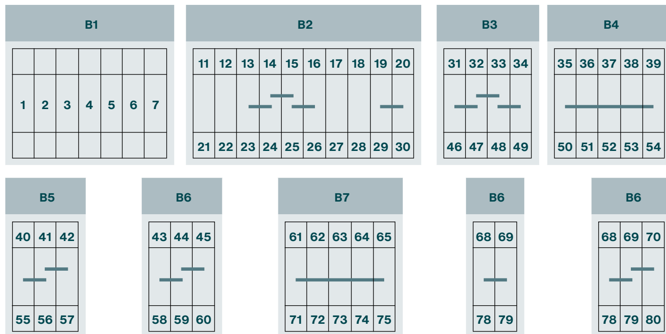
Borniers de la platine de régulation
