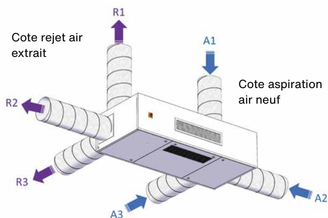
Combinaisons possibles des piquages d'aspiration air neuf et de rejet d'air extrait
