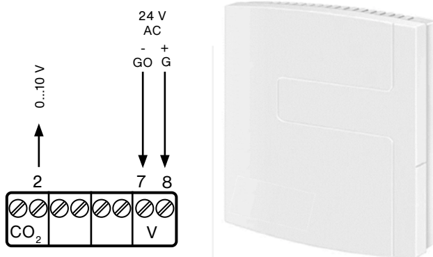
Représentation visuelle de la sonde de CO2 et des bornes de raccordement électrique
